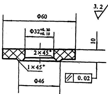
图 1 施载圈
